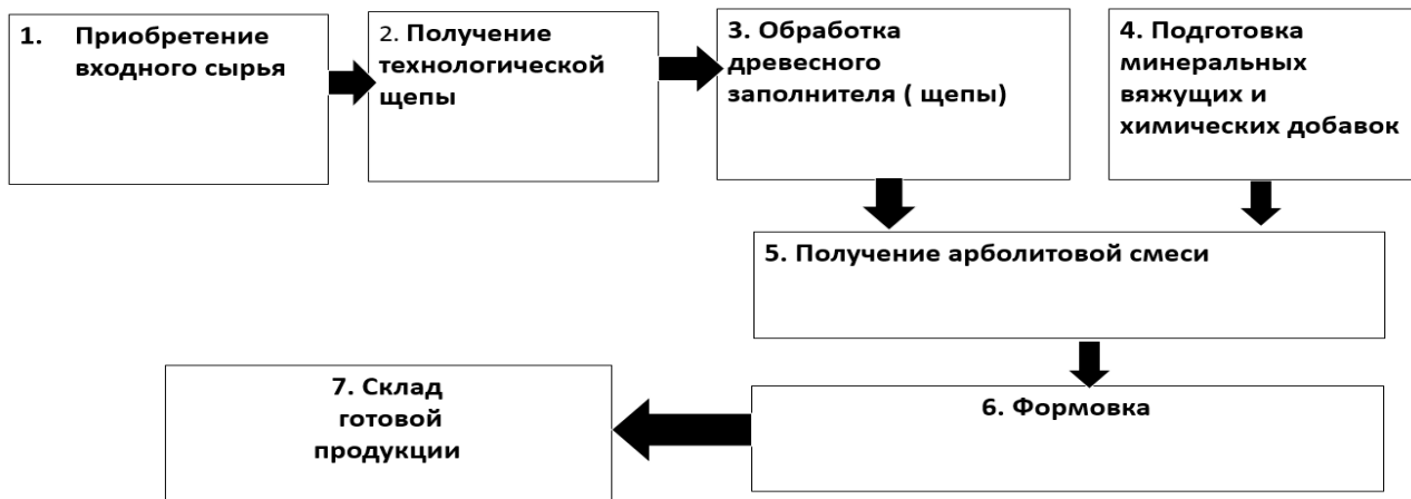
Рис. 1. Производственно-технологическая схема производства арболита
