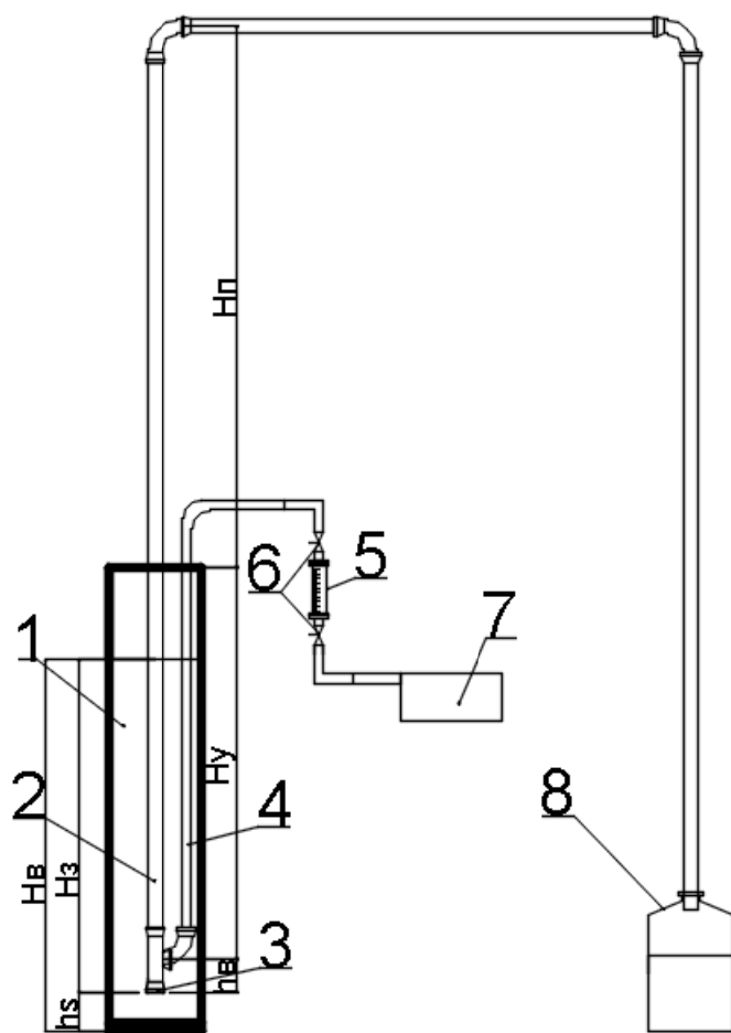
Рис. 3. Схема лабораторной установки где: H_v -уровень воды, H_z -заглубление всаса под уровень воды, h_c -уровень всаса над дном, h_v - разница между всасом и трубой подачи воздуха; H_y + H_p -высота подъёма водо-воздушной смеси; 1-накопительная ёмкость; 2-вертикальная перекачивающая труба; 3-всасывающий оголовок; 4-воздушный патрубок; 5-ротаметр регулирующий расход воздуха; 6-вентили для регулирования расхода воздуха; 7-воздушный компрессор; 8-мерная ёмкость
