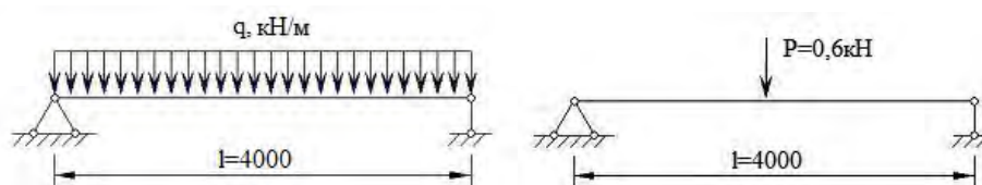
Рис. 2. Расчетные схемы балки при расчете: а) на прочность и прогиб; б) на зыбкость
