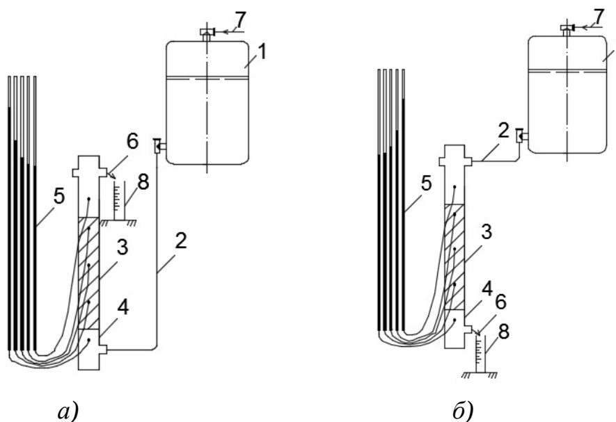
Рис. 1 Схема установки:
