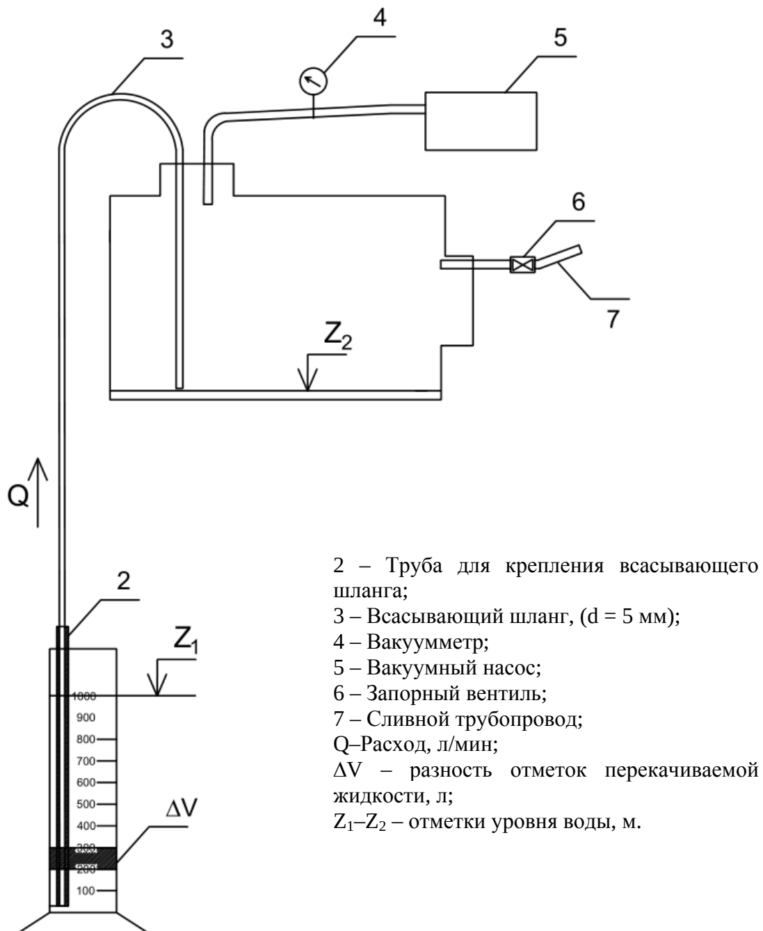
Рис. 1. Чертеж установки
