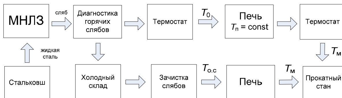
Рис. 1. Схема движения слабов после МНЛЗ
