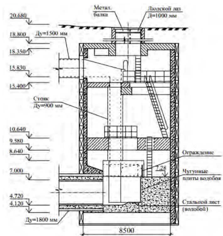
Рис. 1. Канализационная перепадная Шахта №123. Стелками показано направление движения воздуха в пределах сооружения
